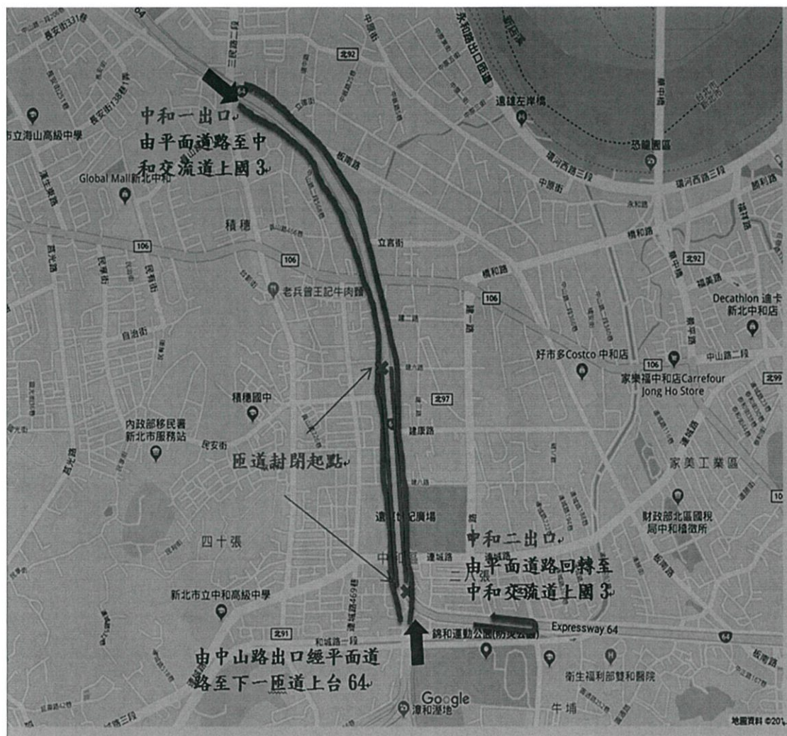
國道3號中和交流道銜接台64線出口及入口匝道改道示意圖
