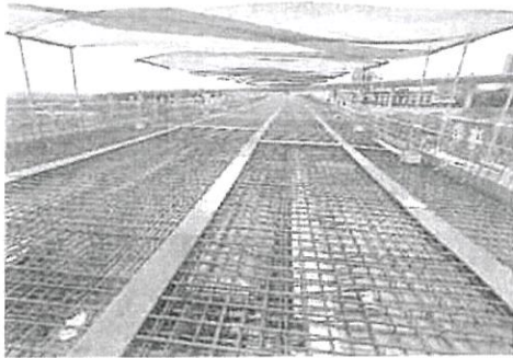
圖 2 架設遮陽網
